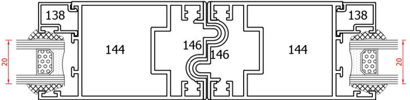
DETAY - 5
