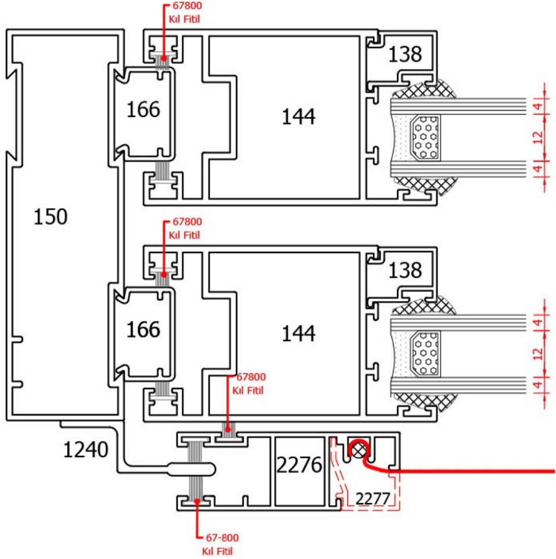
DETAY - 4
