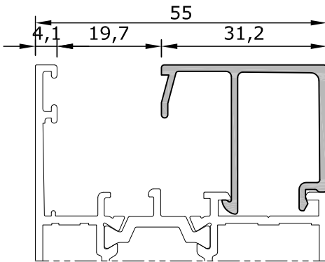
9050 31,2 mm Cam Çıtası 0,360 kg/m
