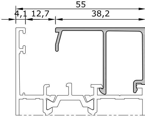
9071 38,2 mm Cam Çıtası 0,385 kg/m
