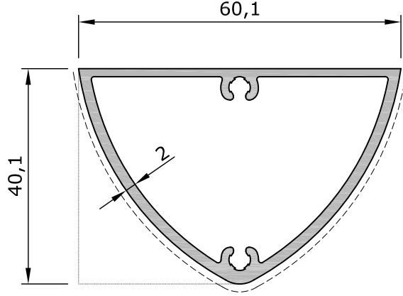
9142 Orta Kayıt Takviye Profili 0,865 kg/m Reinforced Profile for Transom
