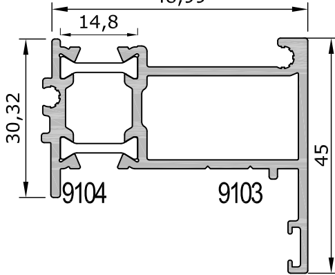
55-9103/9104 Dışa Ağır Hemyüz Çift Kanat Adaptörü 1,065 kg/m Outside Opening Door Adapter
