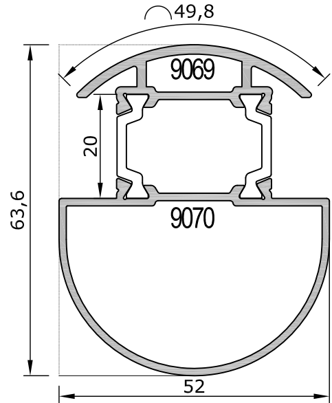
55-9069/9070 Açılı Dönüş Profili 1.250 kg/m | Corner Profile Jx=16,20 cm 4 | Jy=9,14 cm 4
