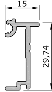
9100 İçe Ağır Hemyüz Kapı Adaptörü 0,295 kg/m Inside Opening Door Adapter
