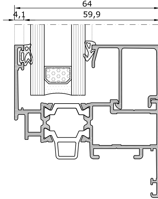
KANAT İÇİN CAM ÇITASI VE FİTİL TABLOSU / GLAZING BEAD AND GASKETS TABLE FOR SASH
