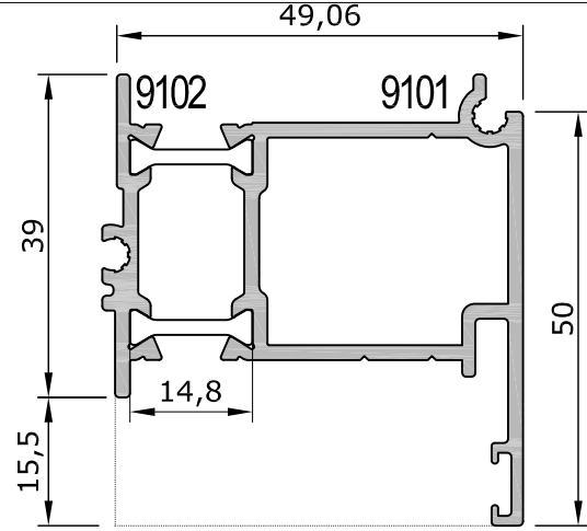
55-9101/9102 Dışa Ağır Hemyüz Kapı Adaptörü 1,195 kg/m Outside Opening Door Adapter
