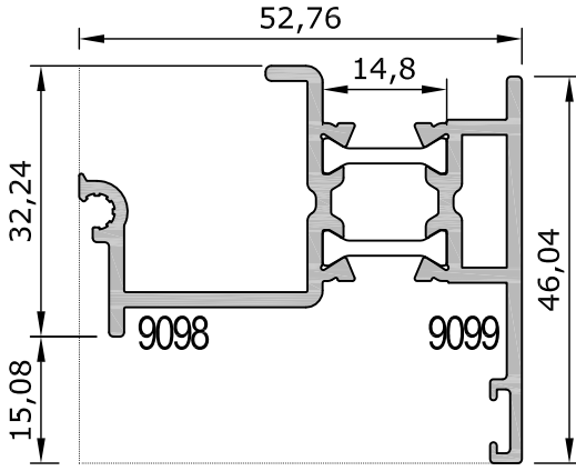
55-9098/9099 İçe Ağır Hemyüz Çift Kanat Adaptörü 1,005 kg/m Inside Opening Door Adapter 48,99
