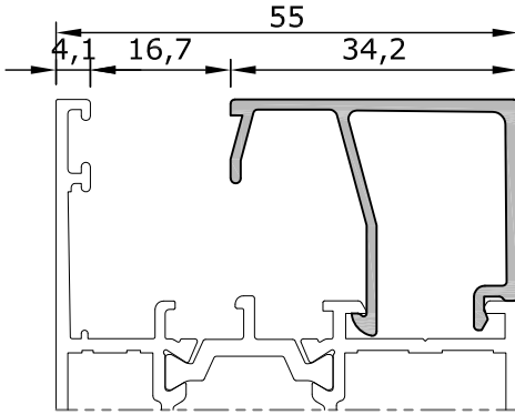
9049 34,2 mm Cam Çıtası 0,370 kg/m
