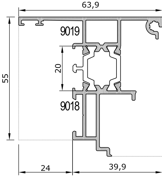
55-9018/9019 Çift Kanat Adaptörü 1.215 kg/m | Double Sash Adapter
